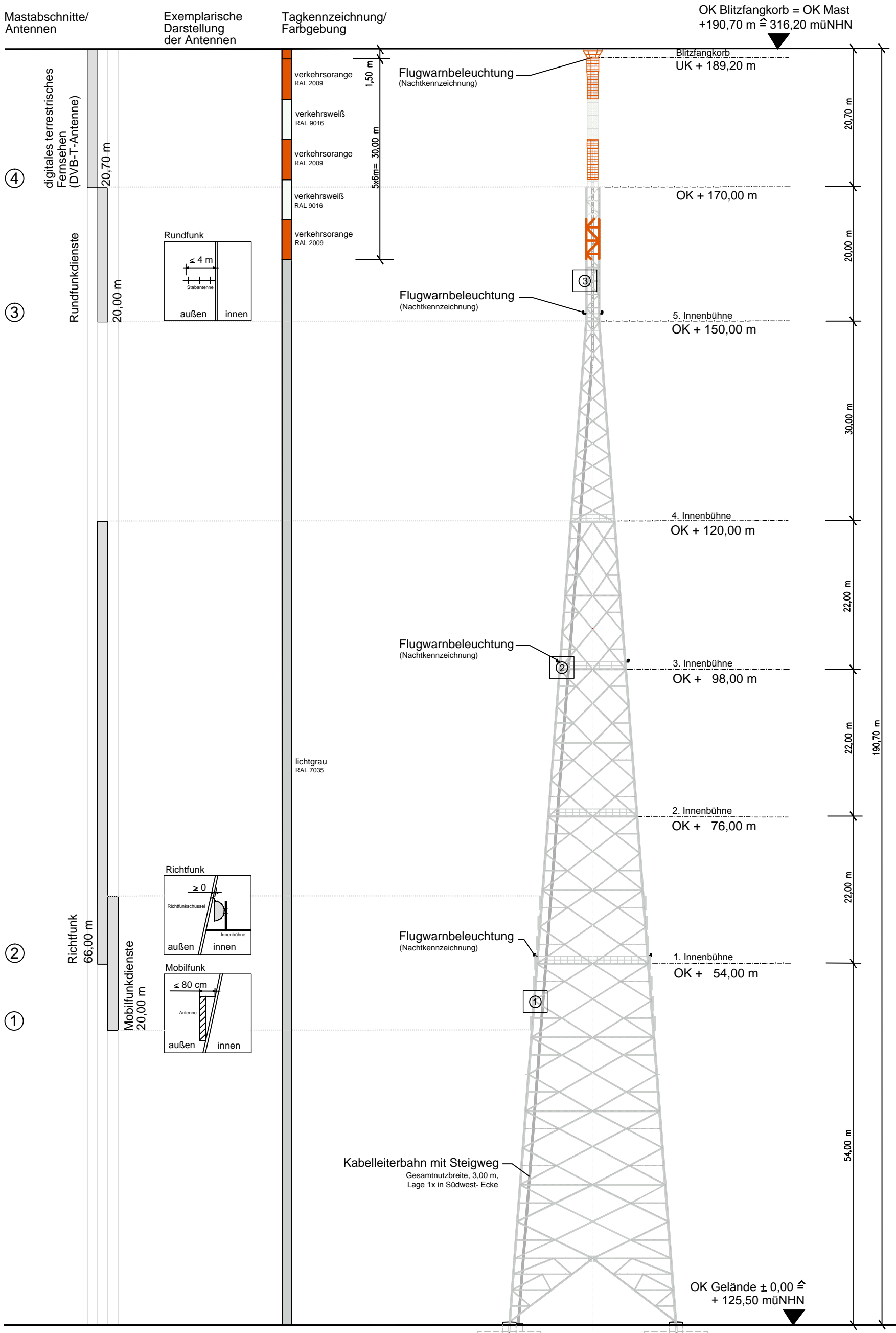
Ansicht von Nord, Ost, Süd und West identisch (außer Kabelleiterbahn, hier Ansicht von Süd)
